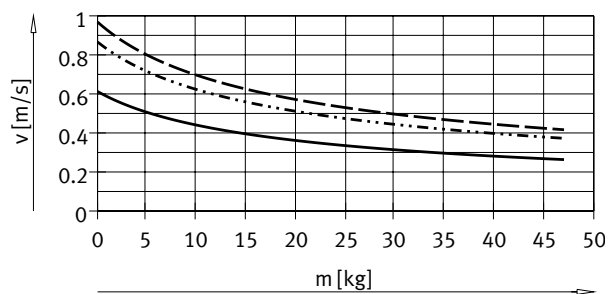
采用缓冲 PPS 时，平均活塞速度 v 与有效负载 m 的关系
