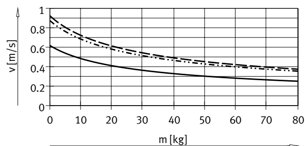
缸径 \varnothing 63
